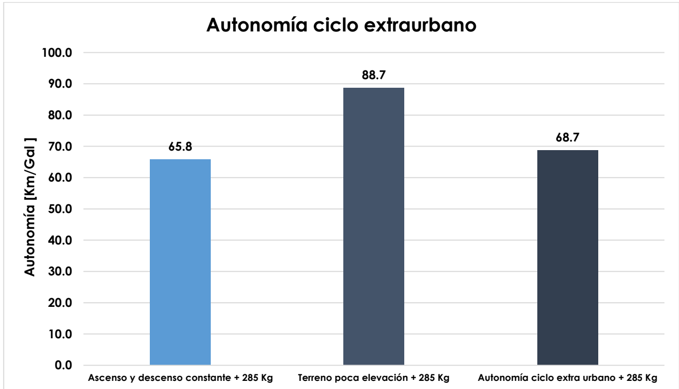
Ilustración 12. Autonomía ciclo extraurbano
