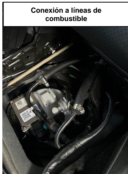
Ilustración 11. Equipo de medición y conexión del equipo a las líneas de combustible.
